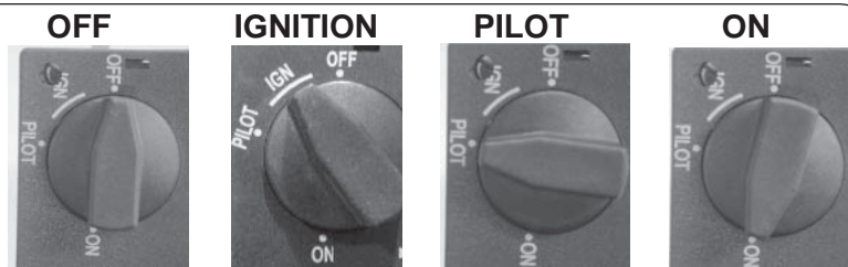
POSITIONS D'OPÉRATION DE CLAPET À GAZ Fig. 14-1
